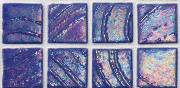
Masaya
