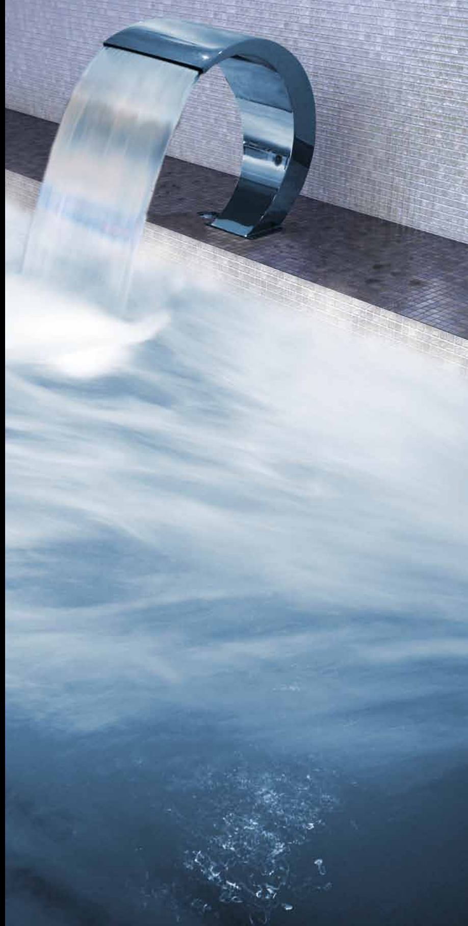
Colima
