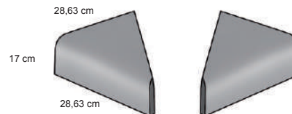
▲ STEP - L ÁNGULO EXTERIOR* 28,63 x 28,63 x 17 cm
