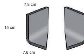
▲ COVEBASE ÁNGULO INTERIOR* 15 x 7,8 x 7,8 cm
